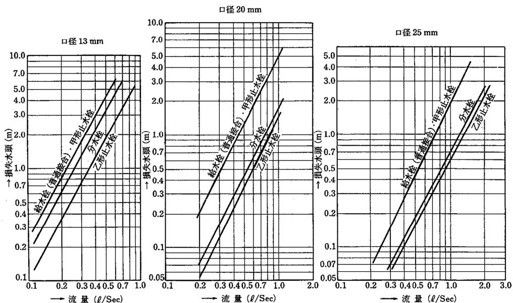
図-11 各種給水用具の標準使用水量に対応する損失水頭
